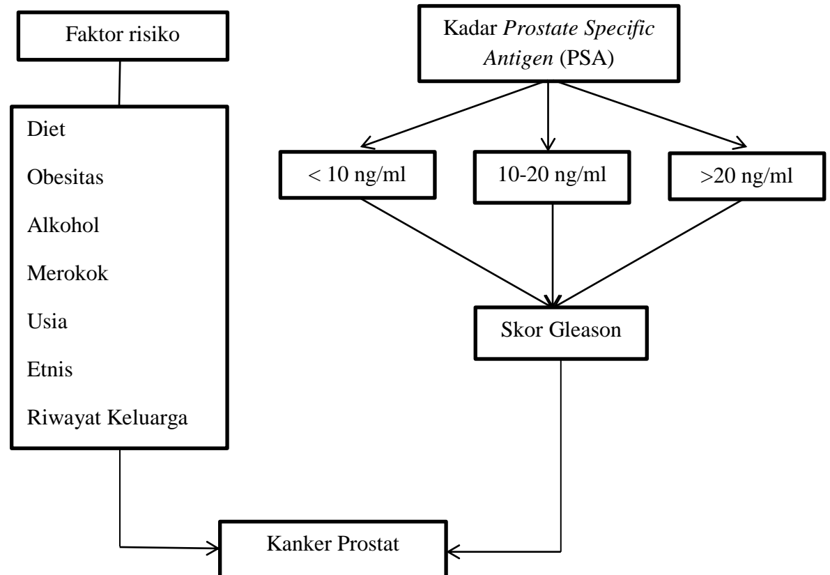
Gambar 2.3 Kerangka Teori
