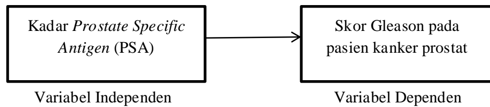
Gambar 2.4 Kerangka Konsep
