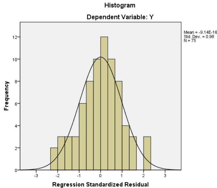
Gambar 4.1 Hasil Grafik Histogram
