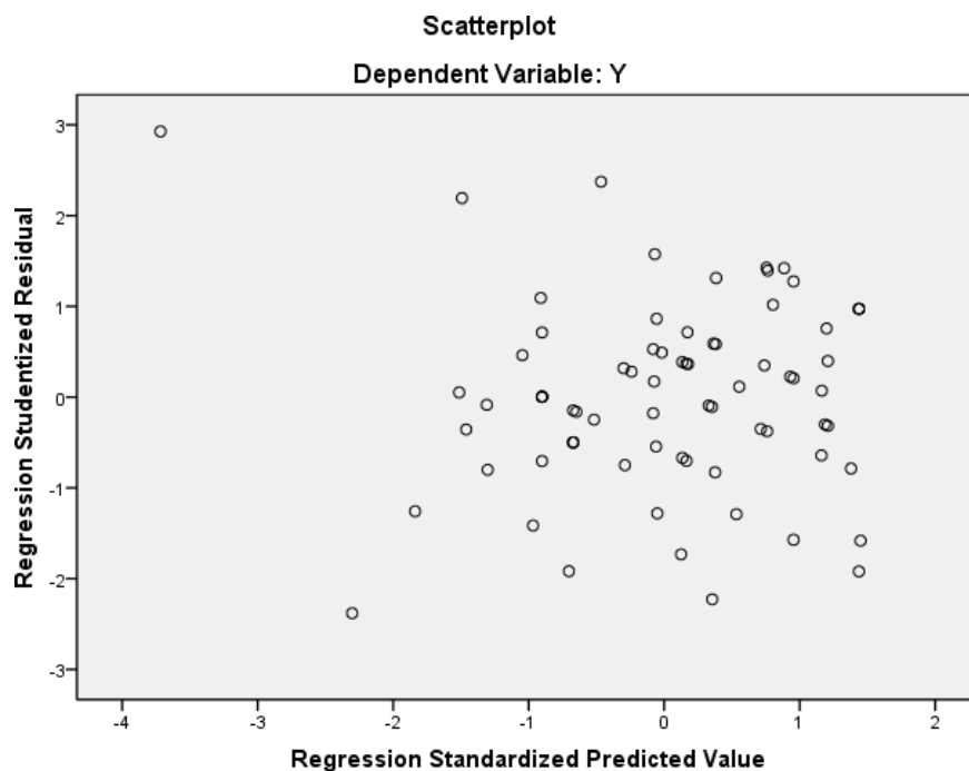
Gambar 4.2 Hasil Grafik Scatterplot
