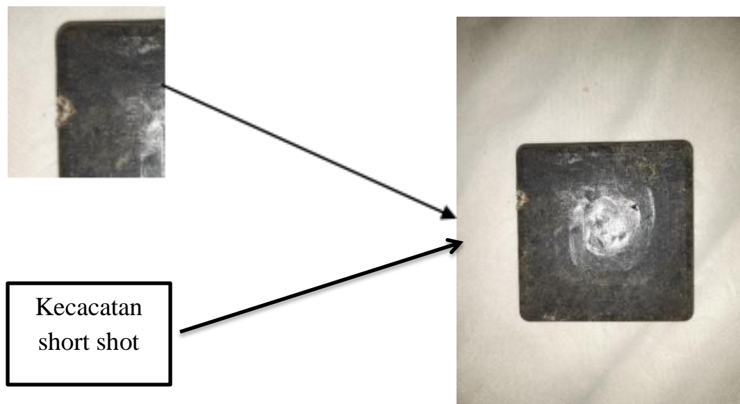
Gambar 4.17 Spesimen pengujian ketiga suhu 200^{\circ}\text{C}
