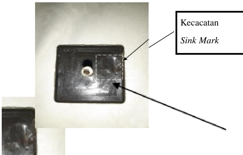
Gambar 4.9 Spesimen pengujian pertama suhu 180°C
