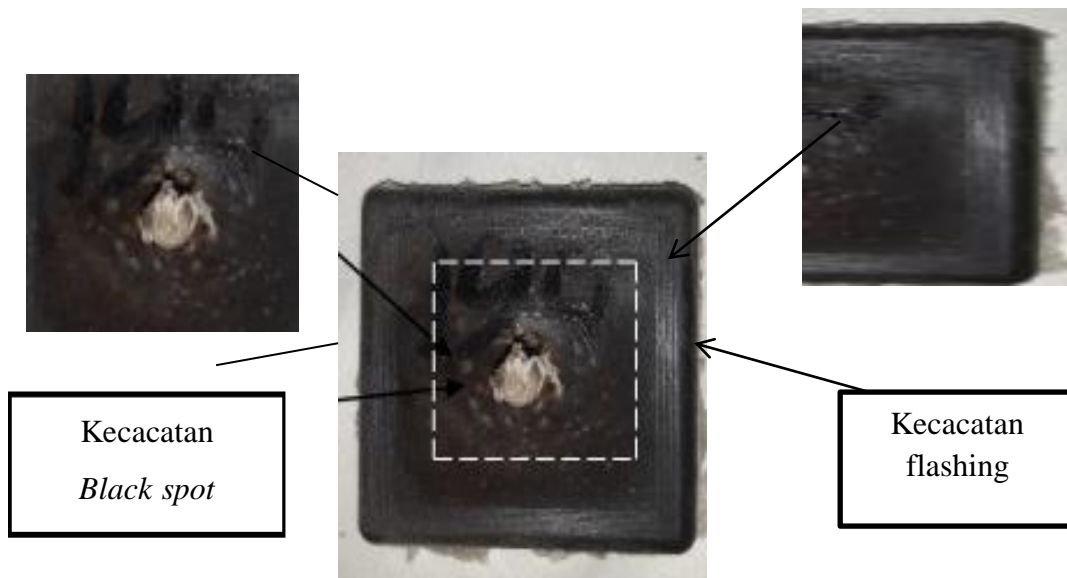
Gambar 4.13 Spesimen pengujian kedua suhu 190°C
