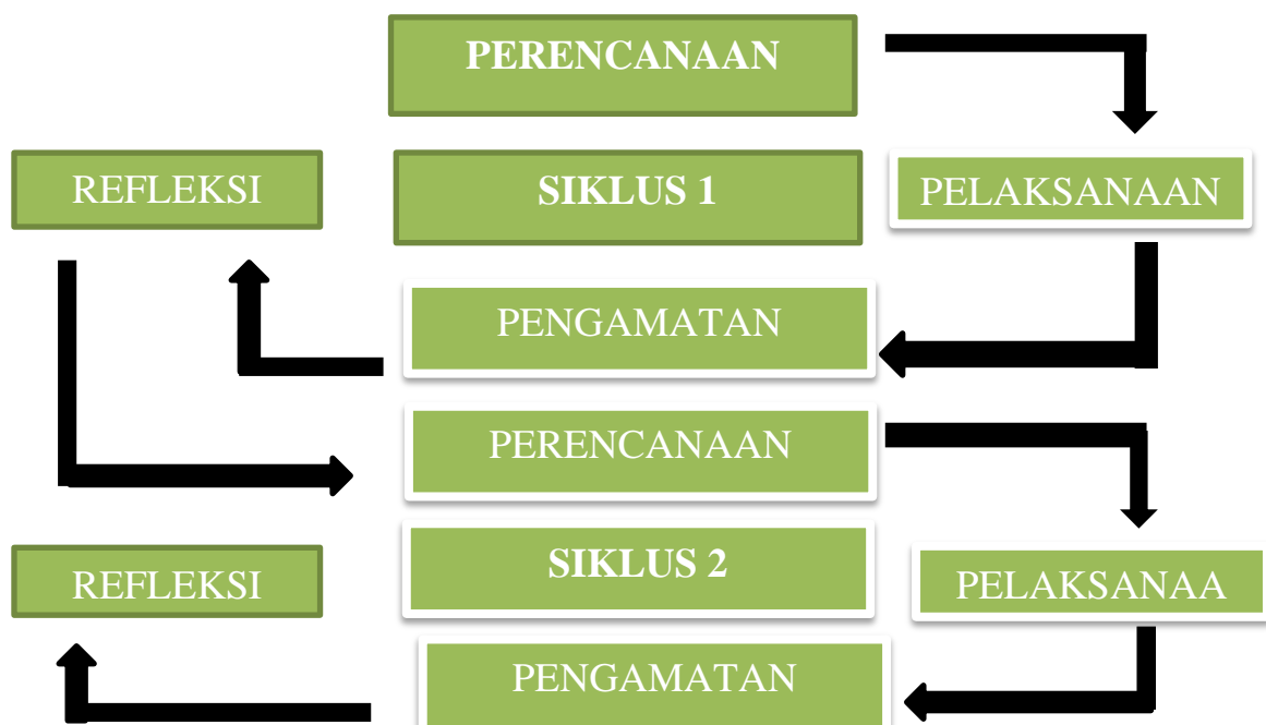
Gambar 3.1 Desain Penelitian
