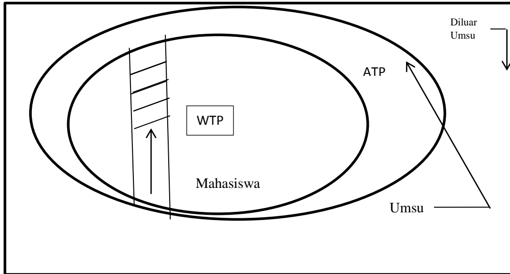
Gambar 2.4: Himpunan ATP
