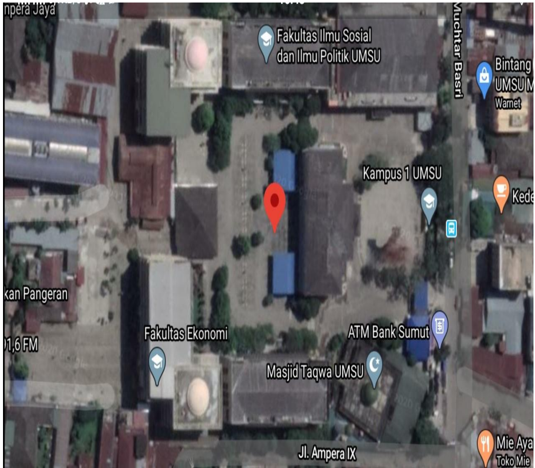
Gambar L2: Lokasi Penelitian
