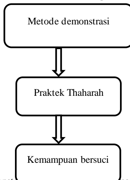
Gambar. 1 Kerangka Berfikir
