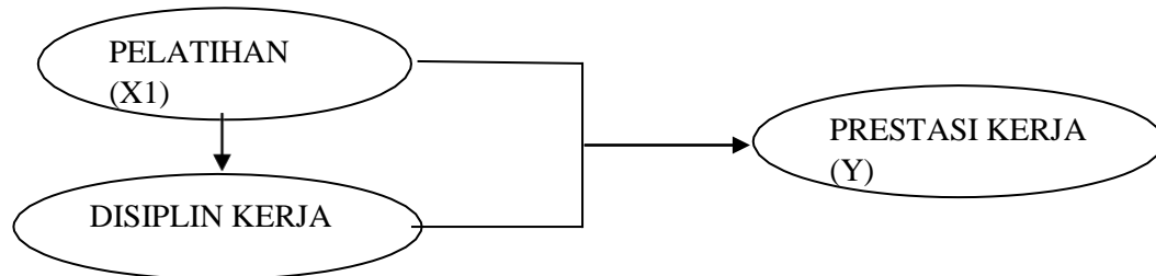
Gambar II.4 Kerangka Konseptual
