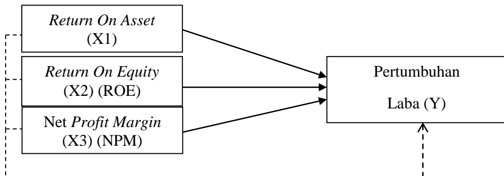
Gambar 2.2 Kerangka Konseptual
