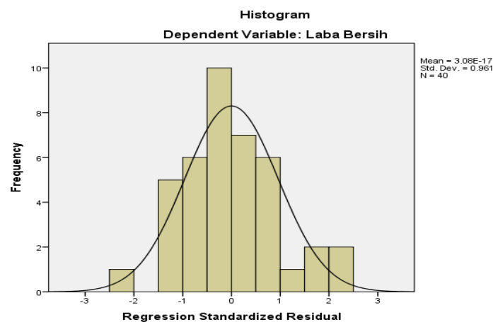
Gambar 4.1 Grafik Histogram
