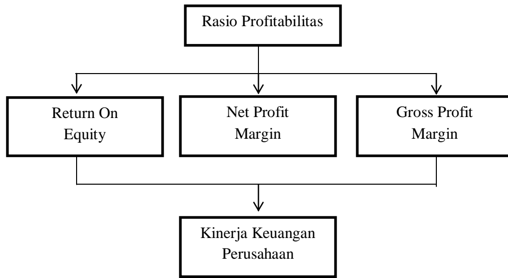
Gambar II.1 Kerangka Berpikir
