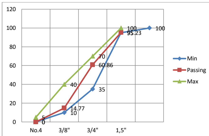
Gambar 3.3: Grafik gradasi agregat kasar diameter maksimum 40 mm.
