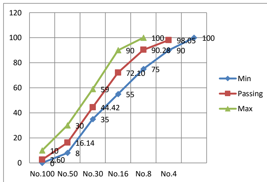
Gambar 3.2: Grafik gradasi agregat halus (zona 2 pasir sedang).
