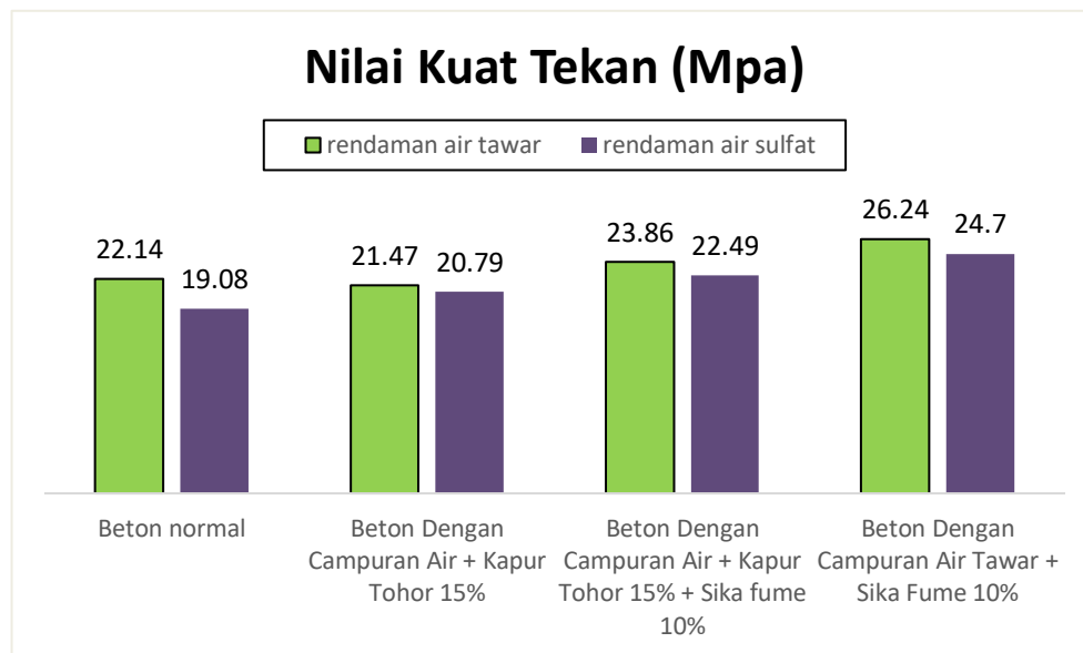
Gambar 4.8: Grafik persentase perbandingan nilai rata-rata kuat tekan beton umur 28 hari rendaman air tawar dan air sulfat.
