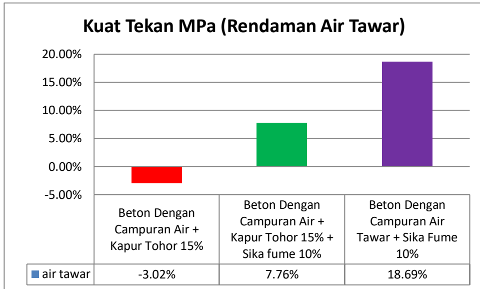
Gambar 4.9: Grafik persentase perbandingan nilai kenaikan rata-rata kuat tekan beton umur 28 hari rendaman air tawar dan air sulfat.
