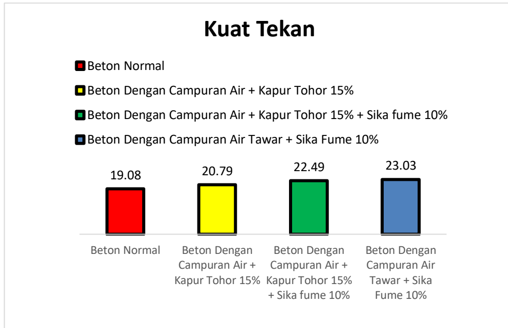
Gambar 4.7: Grafik persentase nilai kuat tekan beton umur 28 hari rendaman air sulfat.
