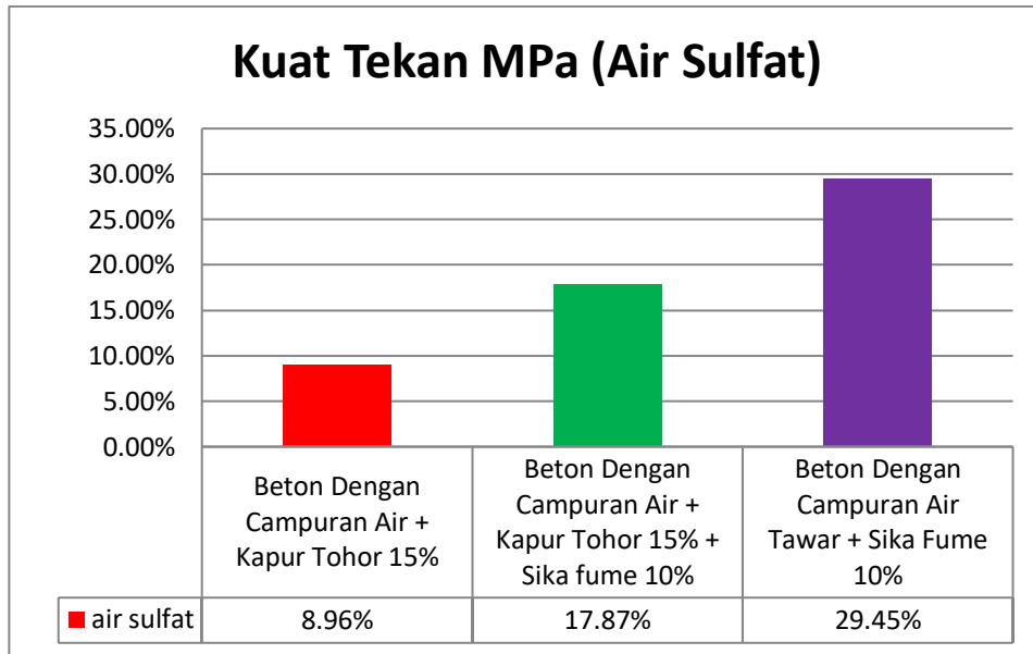
Gambar 5.0: Grafik persentase perbandingan nilai kenaikan rata-rata kuat tekan beton umur 28 hari rendaman air tawar dan air sulfat.
