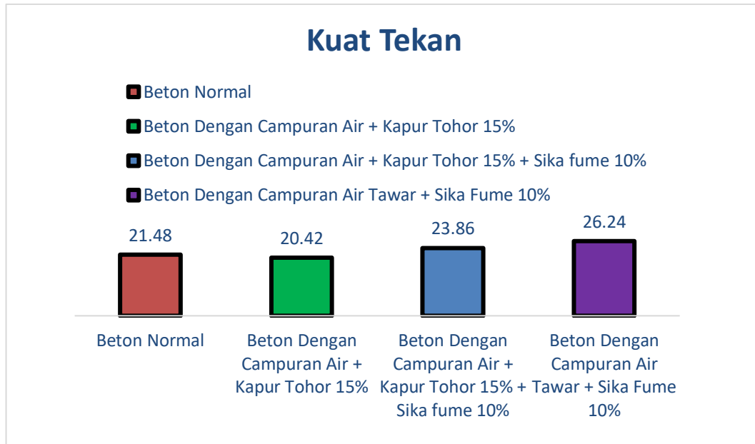
Gambar 4.6: Grafik persentase nilai kuat tekan beton umur 28 hari rendaman air tawar
