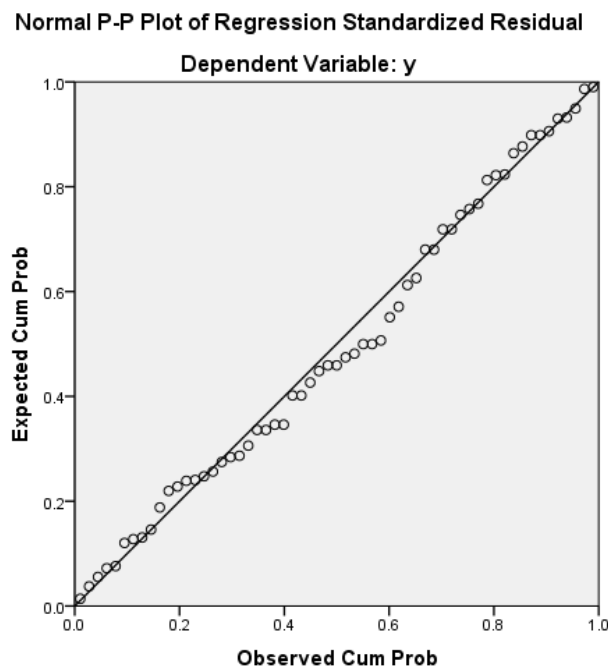
Gambar IV.5 Penelitian menggunakan P-Plot
