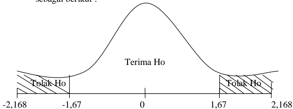
Gambar IV.7 Kurva Distribusi Hipotesis
