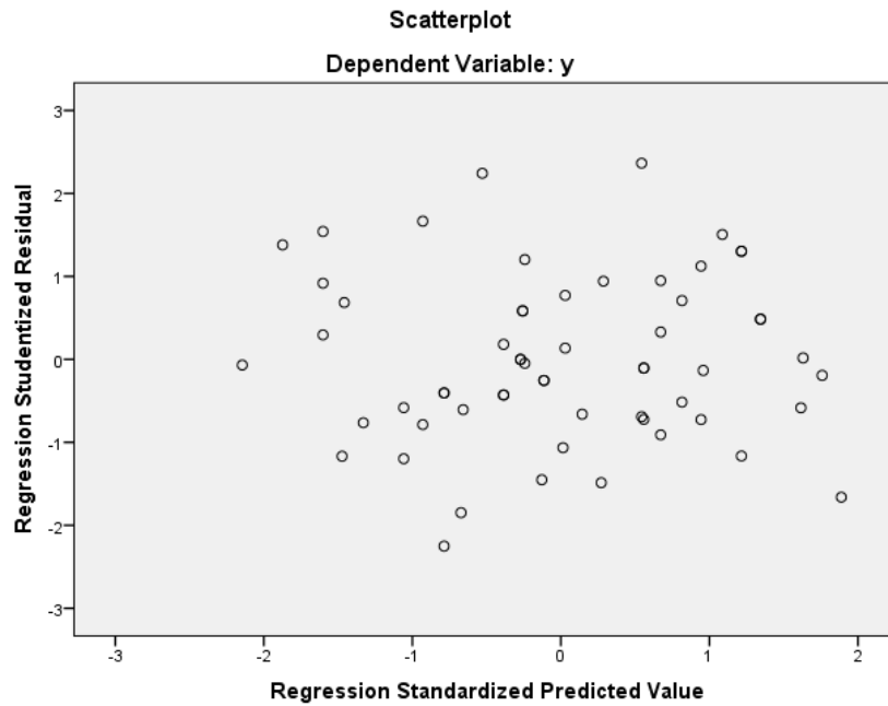
Gambar IV.6 Uji Heterokedastisitas
