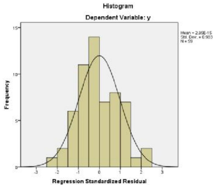
Gambar IV.4 Grafik Histogram
