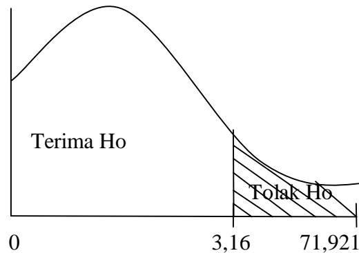
Gambar IV.9 Kurva Distribusi Hipotesis
