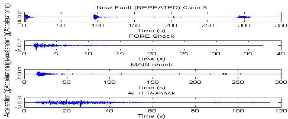
Gambar 3.12: Rekaman gempa Nocera ( fore-shock ), niigata Japan ( main-shock ), dan niigata Japan ( after-shock ) setelah digabungkan ( near-fault Repeated ), ini termasuk gempa berulang 3 kali.
