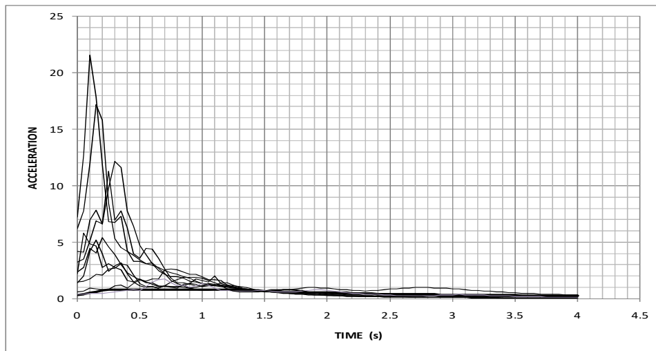
Gambar 3.9: Respon spektrum dengan 10 daerah gempa setelah diskalakan terhadap respon spektrum diindonesia (Banda Aceh).
