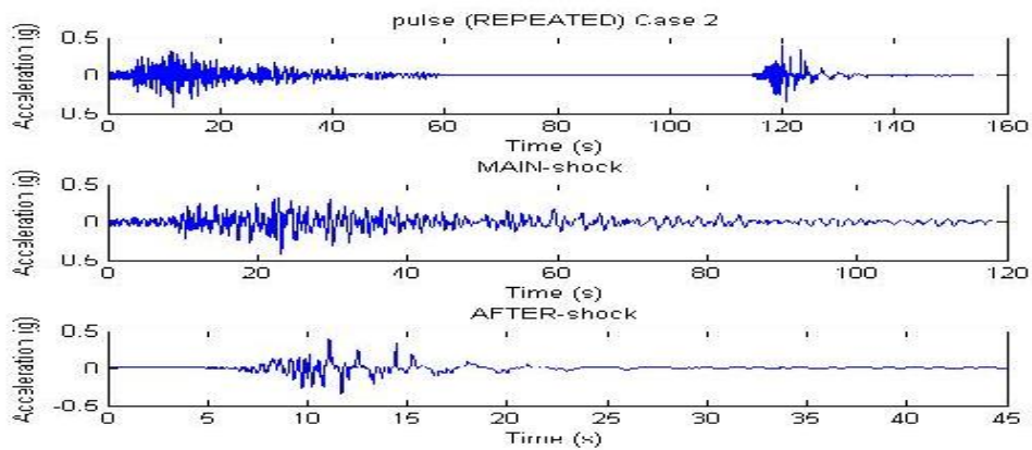
Gambar 3.11: Rekaman gempa Hokkaido Japan ( Main-shock ) dan Christchurch New Zealand ( after-shock ) setelah digabungkan ( pulse Repeated ), ini termasuk gempa berulang 2 kali.
