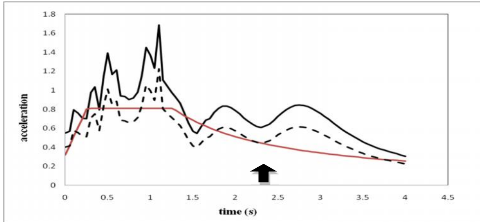
Gambar 3.8: Respon spektrum Christchurch New Zealand setelah diskalakan (garis putus-putus) terhadap respon spektrum diindonesia (Banda Aceh).
