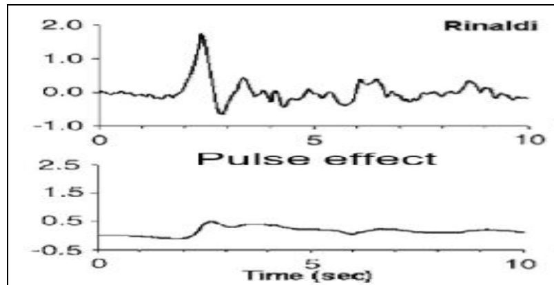
Gambar 2.3: Rekaman gempa Northridge (1994) dan Parkfield (1997) (Pawirodikromo, 2012).
