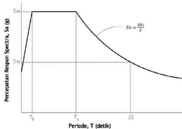
Gambar 2.7: Spektrum respons desain.
