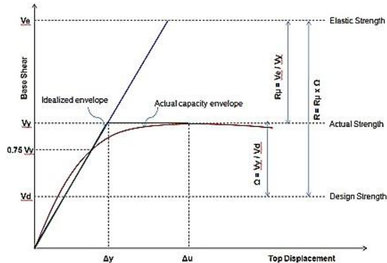
Gambar 2.6: Hubungan antara faktor modifikasi respon ( R ), faktor kuat lebih struktur ( R\mu ), dan faktor reduksi daktilitas ( R\mu )
