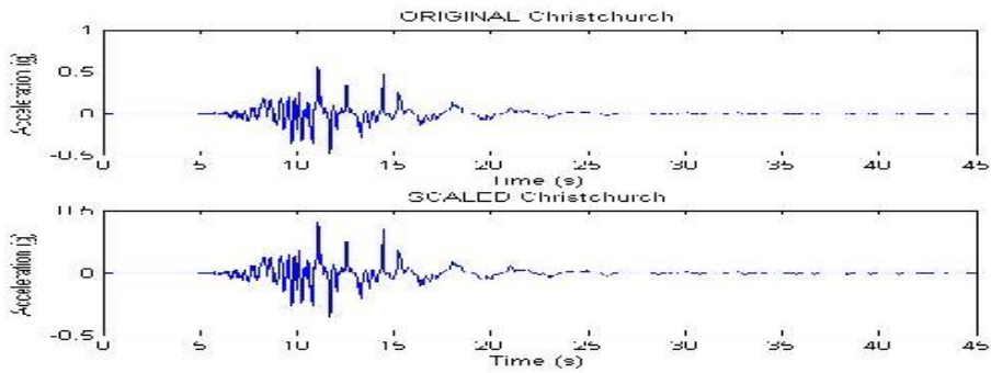
Gambar 3.10: Rekaman gempa Christchurch New Zealand setelah diskalakan (gambar bawah) ini termasuk gempa tunggal.
