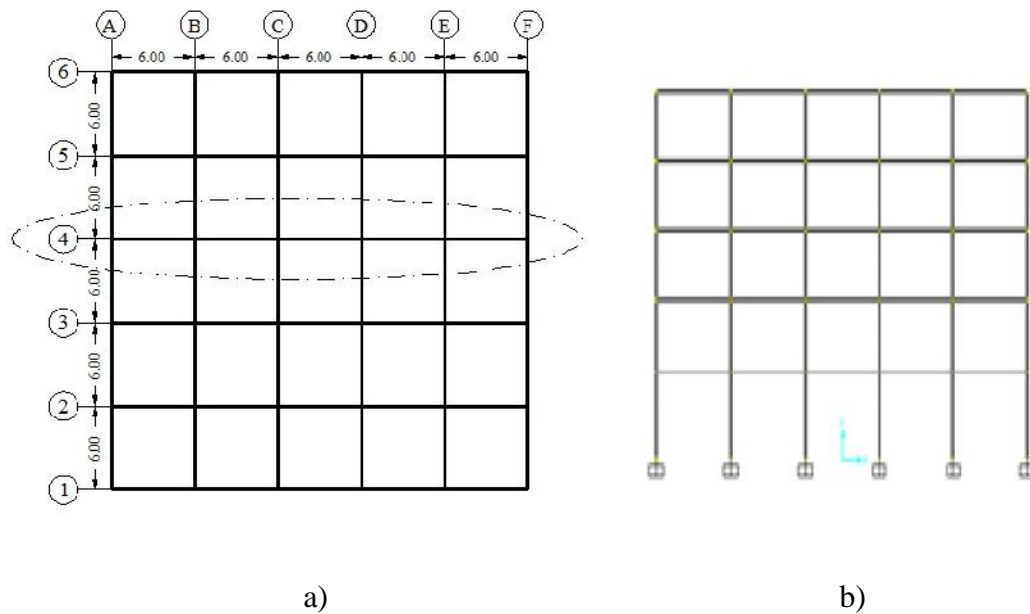
Gambar 3.2: a) Denah struktur Model 1, b) Proyeksi bangunan Model 1, c) Denah struktur Model 2, d) Proyeksi bangunan Model 2, e) Denah struktur Model 3, f) Proyeksi bangunan Model 3, g) Denah struktur Model 4; h) Proyeksi bangunan Model 4., i) Denah struktur Model 5, j) Proyeksi bangunan Model 5.
