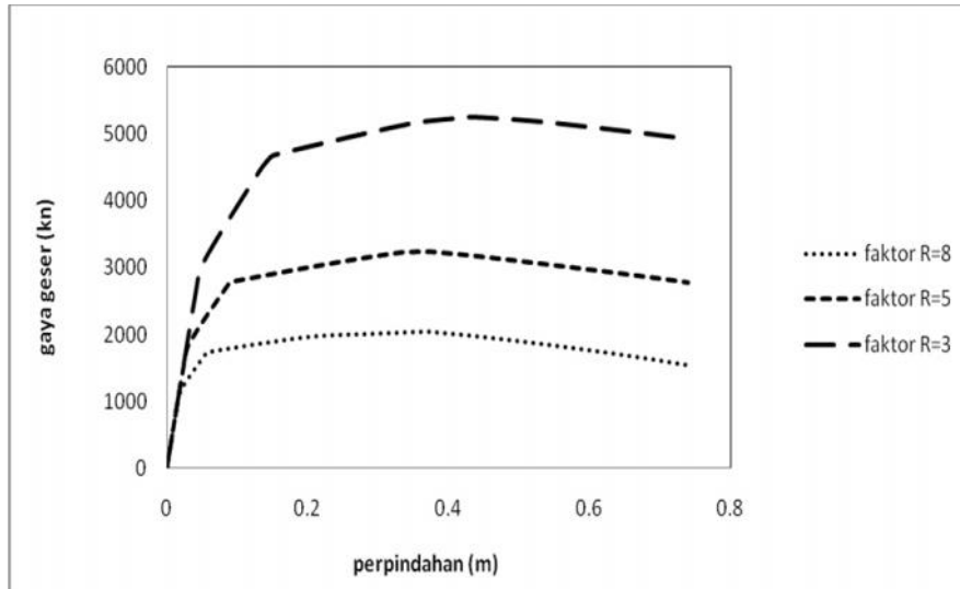
Gambar 3.13: kurva kapasitas untuk ketiga faktor R
