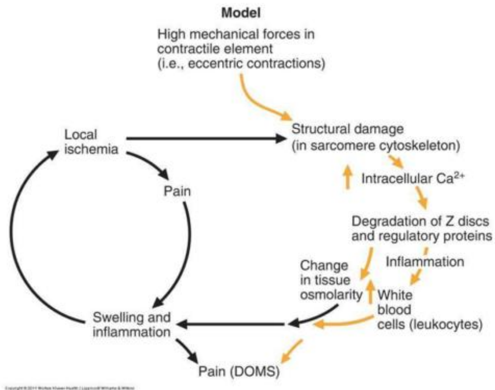
Gambar 2.1 Mekanisme DOMS
