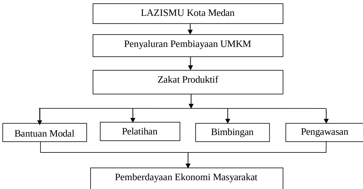
Gambar 2.1 Kerangka Pemikiran
