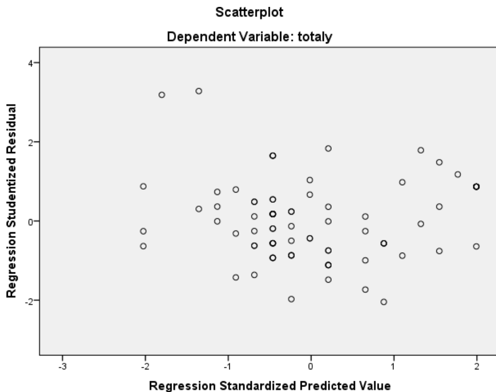
Gambar 4. 3. Uji Heterokedastisitas
