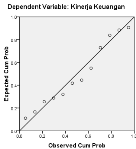
Gambar 4.1 P-plot normalitas
