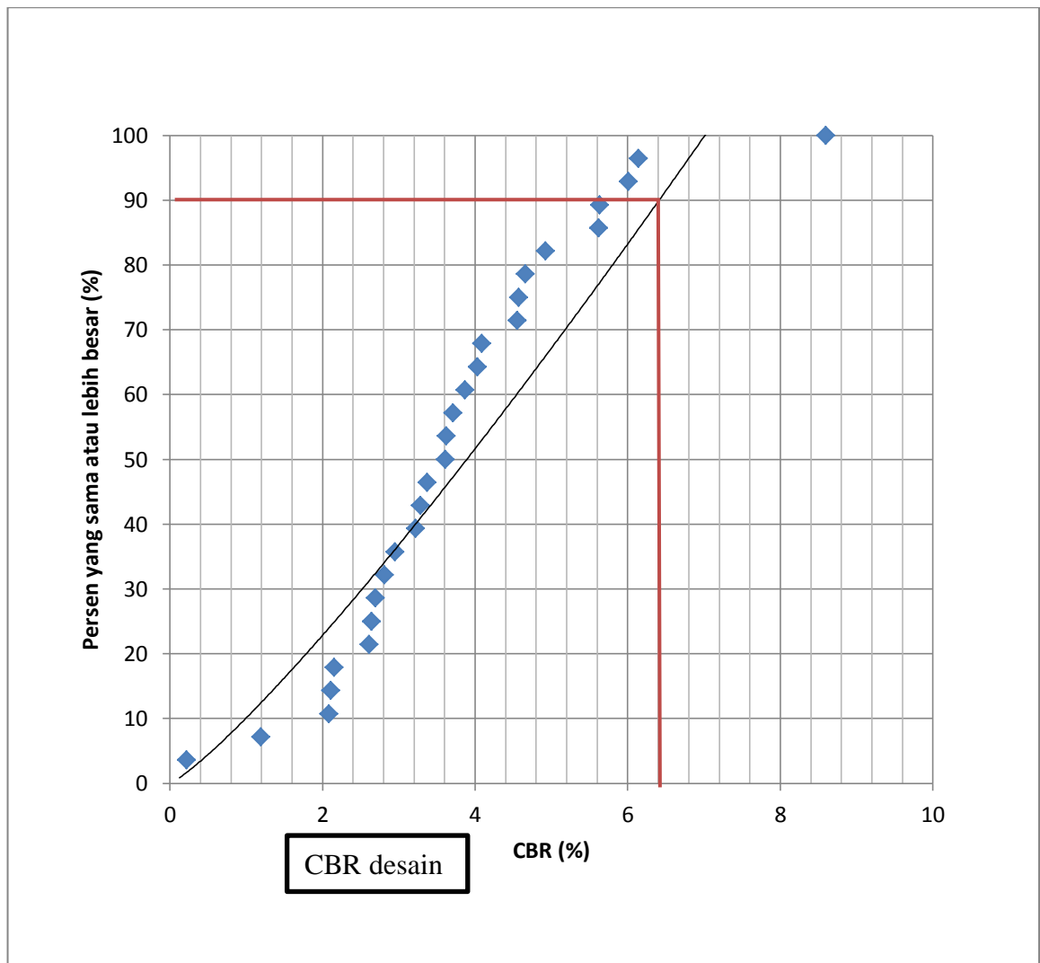
Gambar 4.1: Grafik CBR
