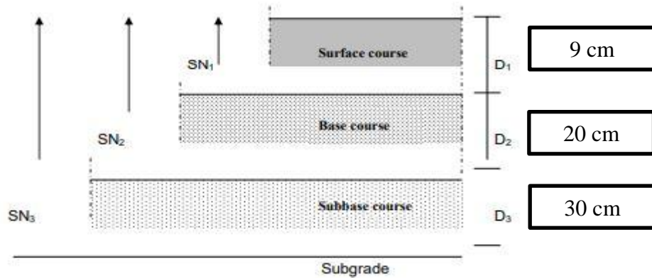
Gambar 4.7: Detail Perkerasan Lapangan
