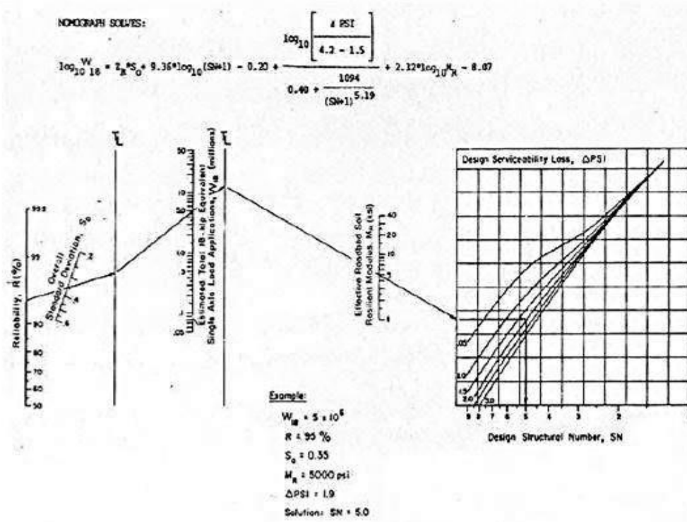
Gambar 2.3: Nomogram untuk menentukan SN perkerasan lentur (Sukirman, 2010)
