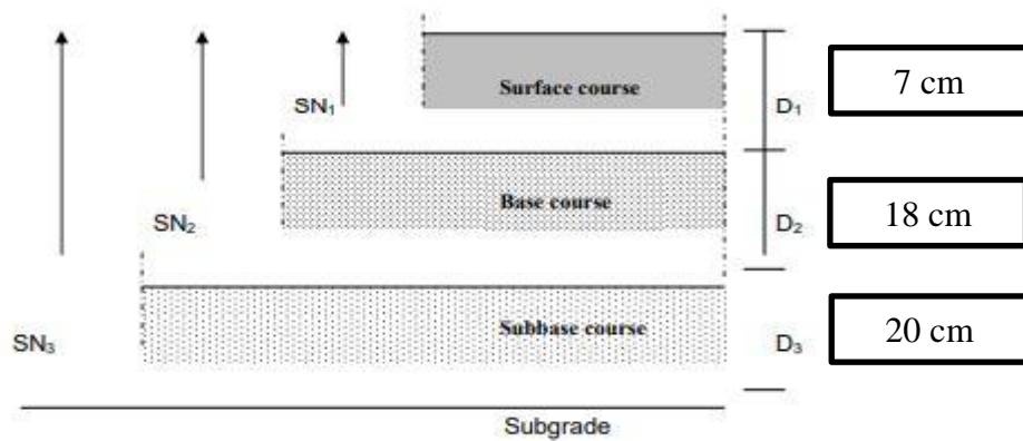
Gambar 4.6: Detail Perkerasan Metode AASHTO 1993
