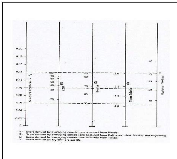
Gambar 2.5: Variasi koefisien lapisan lapis pondasi bawah (Anai et al., 2019)
