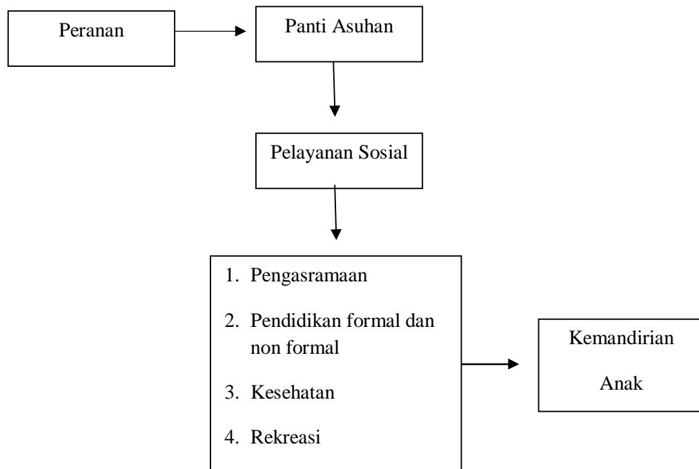
Gambar 1: Kerangka Konsep
