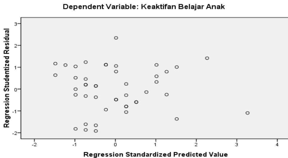
Gambar 4.2 Hasil Uji Heteroskedastisitas Scatterplot
