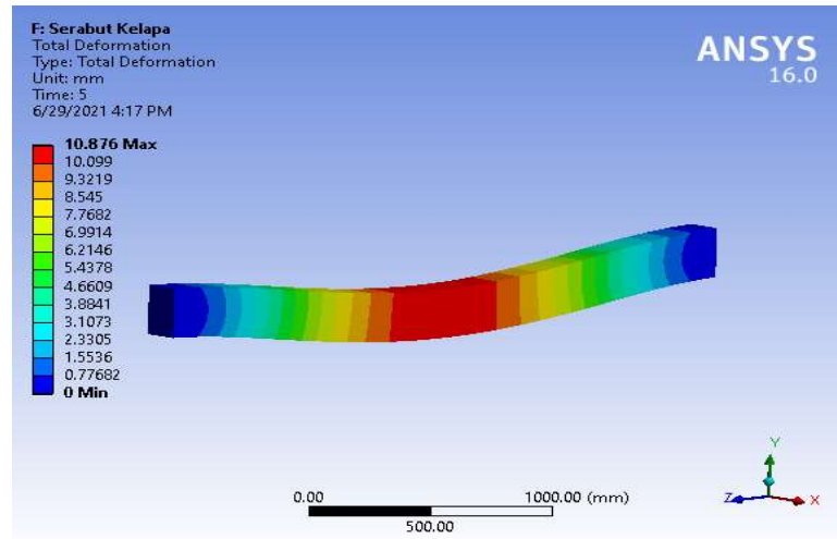
Gambar 4.7: Diagram Kontur Hasil Simulasi Deformasi Balok Beton Dengan Filler Serat Serabut Kelapa.
