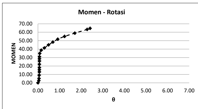
Gambar 4.11: Grafik Hubungan Momen Rotasi Beton Dengan Filler Fly Ash Berdasarkan Ansys
