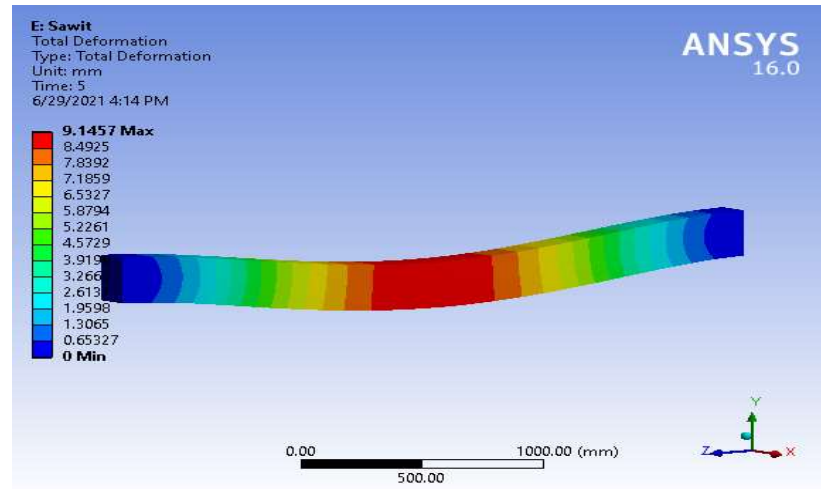
Gambar 4.13: Hasil Deformasi Balok Beton Dengan Filler Serbuk Cangkang Sawit Akibat Gaya Aksial Secara Simulasi
