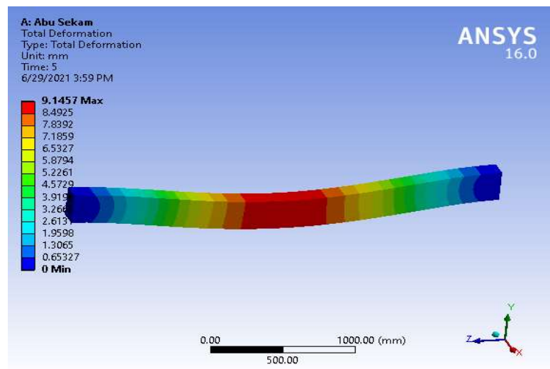
Gambar 4.1: Deformasi Yang Terjadi Pada Balok Beton Dengan Filler Abu Sekam Padi Akibat Gaya Aksial
