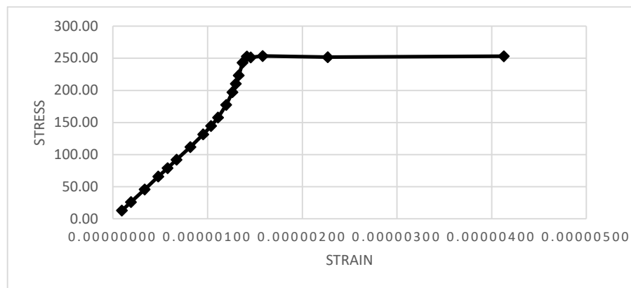
Gambar 4.3: Hubungan Tegangan Regangan Pada Balok Beton Dengan Filler Abu Sekam Padi
