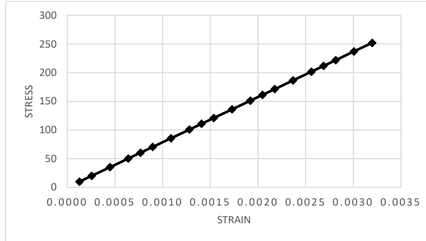
Gambar 4.12: Hubungan Antara Tegangan Dan Regangan Balok Beton Dengan Filler Fly Ash .
