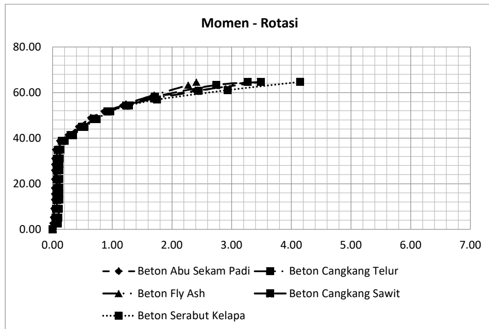
Gambar 4.17: Perbandingan Momen Rotasi Masing-Masing Campuran Beton
