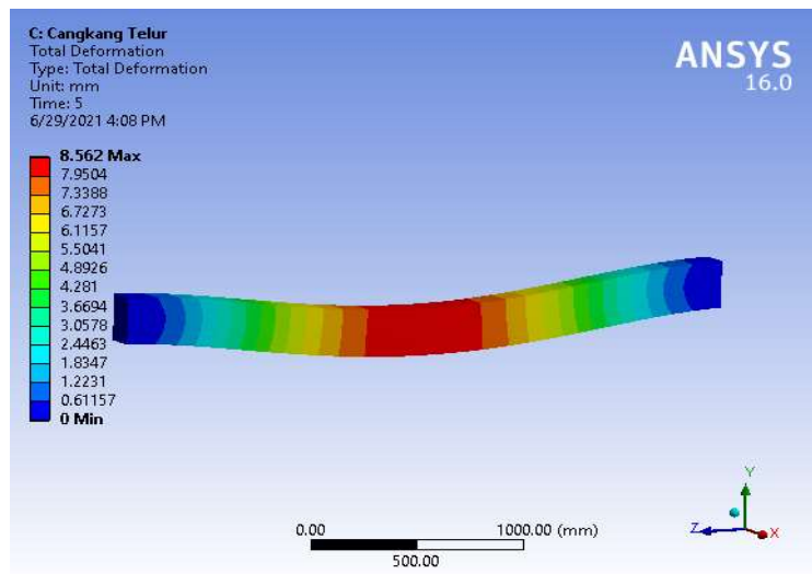
Gambar 4.4: Deformasi Yang Terjadi Pada Balok Beton Dengan Campuran Cangkang Telur
