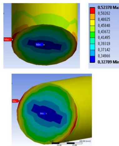
Gambar 2.5: Equivalent Stress Kolom Berdasarkan Pemodelan Ansys
