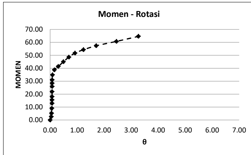
Gambar 4.5: Grafik Hubungan Momen Rotasi Beton Dengan Filler Cangkang Telur Berdasarkan Ansys
