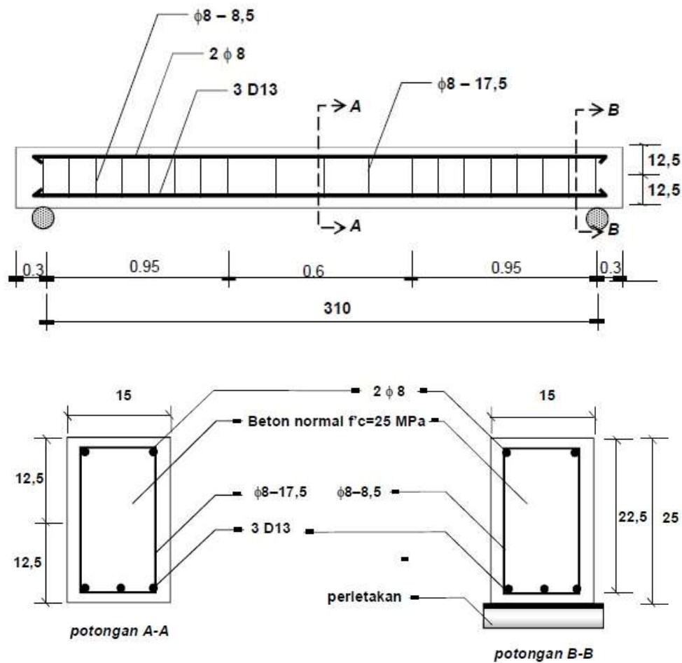
Gambar 2.1: Desain balok beton normal
