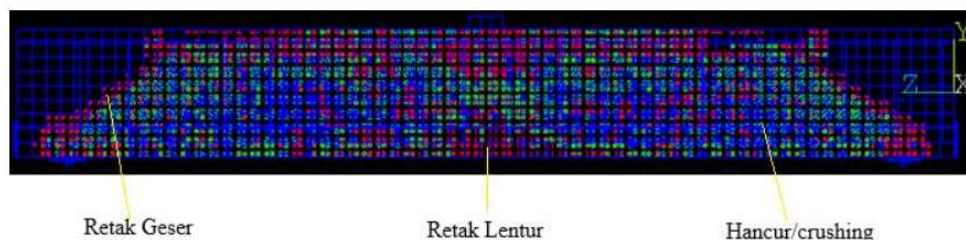
Gambar 2.6: Pola Retak Balok Berdasarkan Pemodelan Ansys
