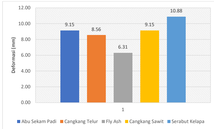
Gambar 4.16: Grafik Perbandingan Hasil Simulasi Material Balok Beton
