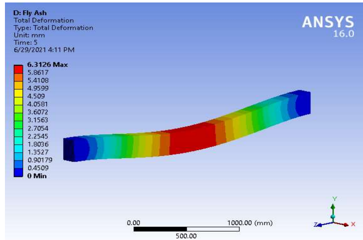
Gambar 4.10: Deformasi Yang Terjadi Pada Baok Beton Dengan Filler Fly Ash Mengakibatkan Gaya Aksial
