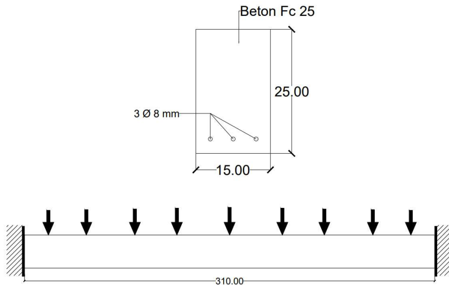
Gambar 3.4: Desain Balok Yang Akan Dilakukan Simulasi
