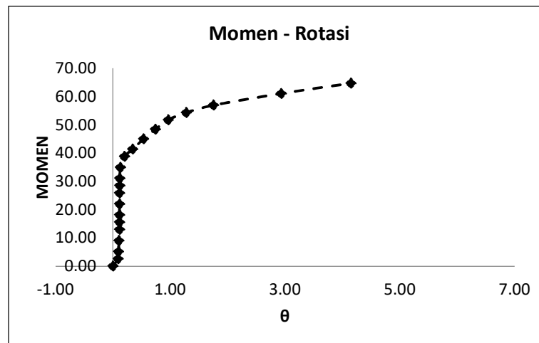
Gambar 4.8: Grafik Hubungan Momen Rotasi Beton Dengan Filler Serabut Kelapa Berdasarkan Ansys
