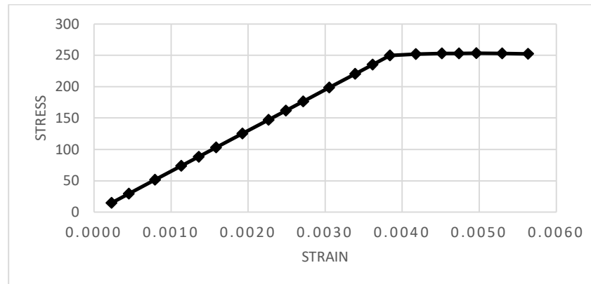
Gambar 4.9: Hubunagn Antara Tegangan Dan Regangan Balok Beton Dengan Filler Serat Serabut Kelapa Mengakibatkan Gaya Aksial
