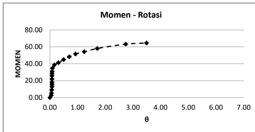
Gambar 4.14: Grafik Hubungan Momen Rotasi Beton Dengan Filler Serbuk Cangkang Sawit Berdasarkan Ansys
