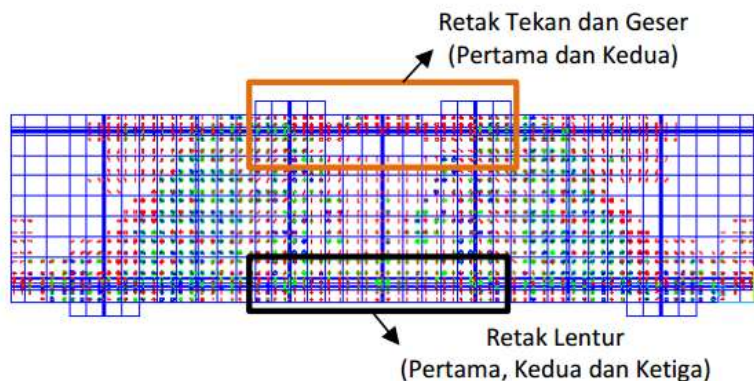
Gambar 2.4: Pemodelan Pola Retak Beton
