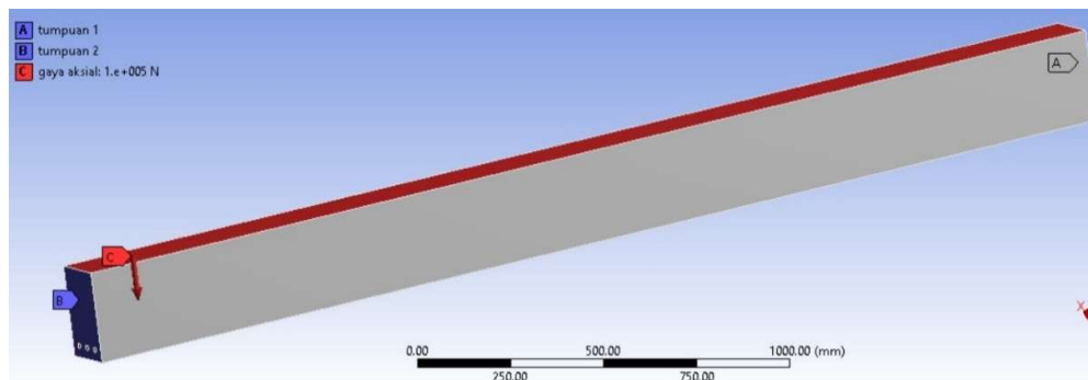
Gambar 3.54: Pengecekan Tumpuan dan Pembebanan
