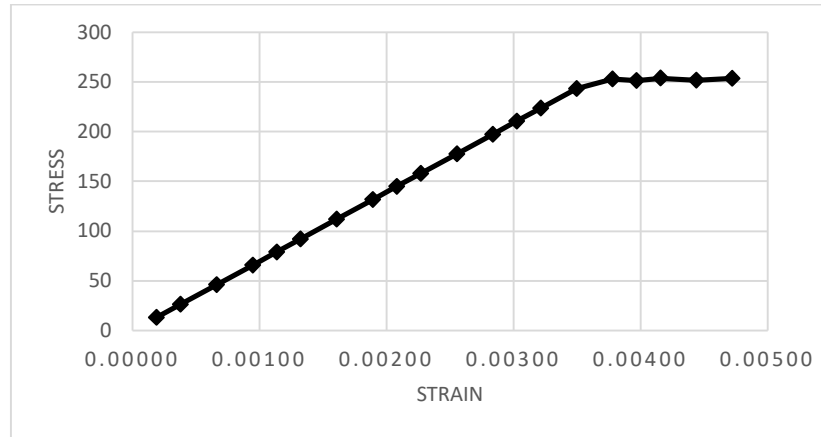
Gambar 4.15: Hubungan Antar Tegangan Dan Regangan Pada Balok Beton Dengan Filler Serbuk Cangkang Sawit
