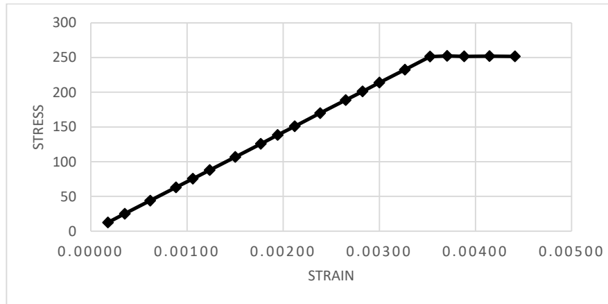
Gambar 4.6: Grafik Hubungan Antara Tegangan Dan Regangan Pada Balok Beton Dengan Filler Serbuk Cangkang Telur
