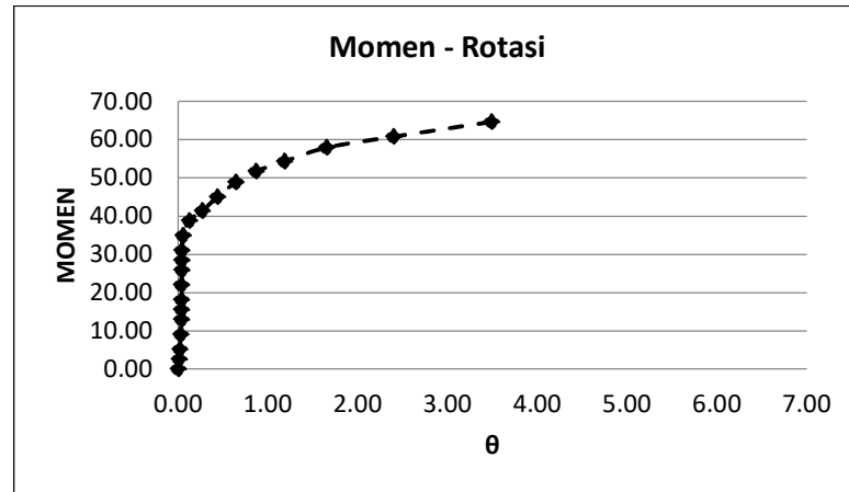
Gambar 4.2: Grafik Hubungan Momen Rotasi Beton Dengan Filler Abu Sekam Padi Berdasarkan Ansys
